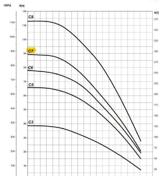
Kapacitetskurva pump SAER C/7 MBS 3,3 kW, 380-415V, 50Hz, 7,2A
