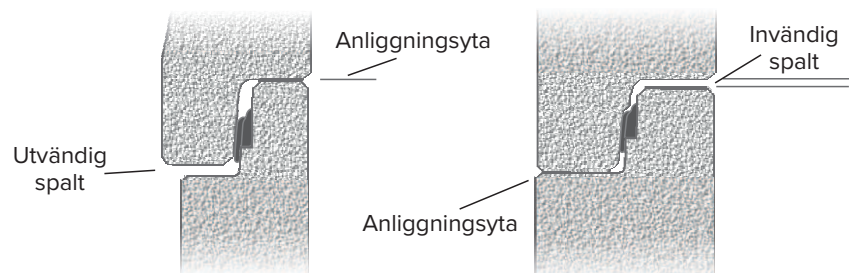
Brunn DN 1600 - 2000 Brunnsringar monterade med glidfogstättning i rätt läge.
